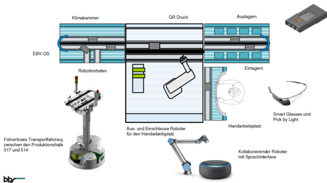
Abbildung 1: Produktionsprozess
