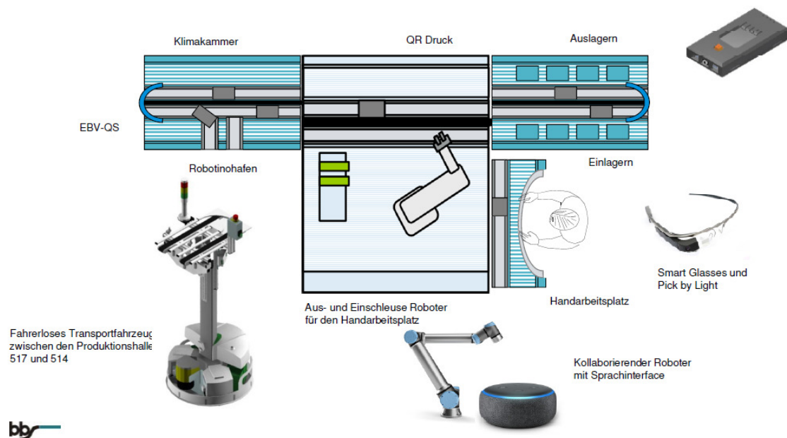
Abbildung 1: Produktionsprozess
